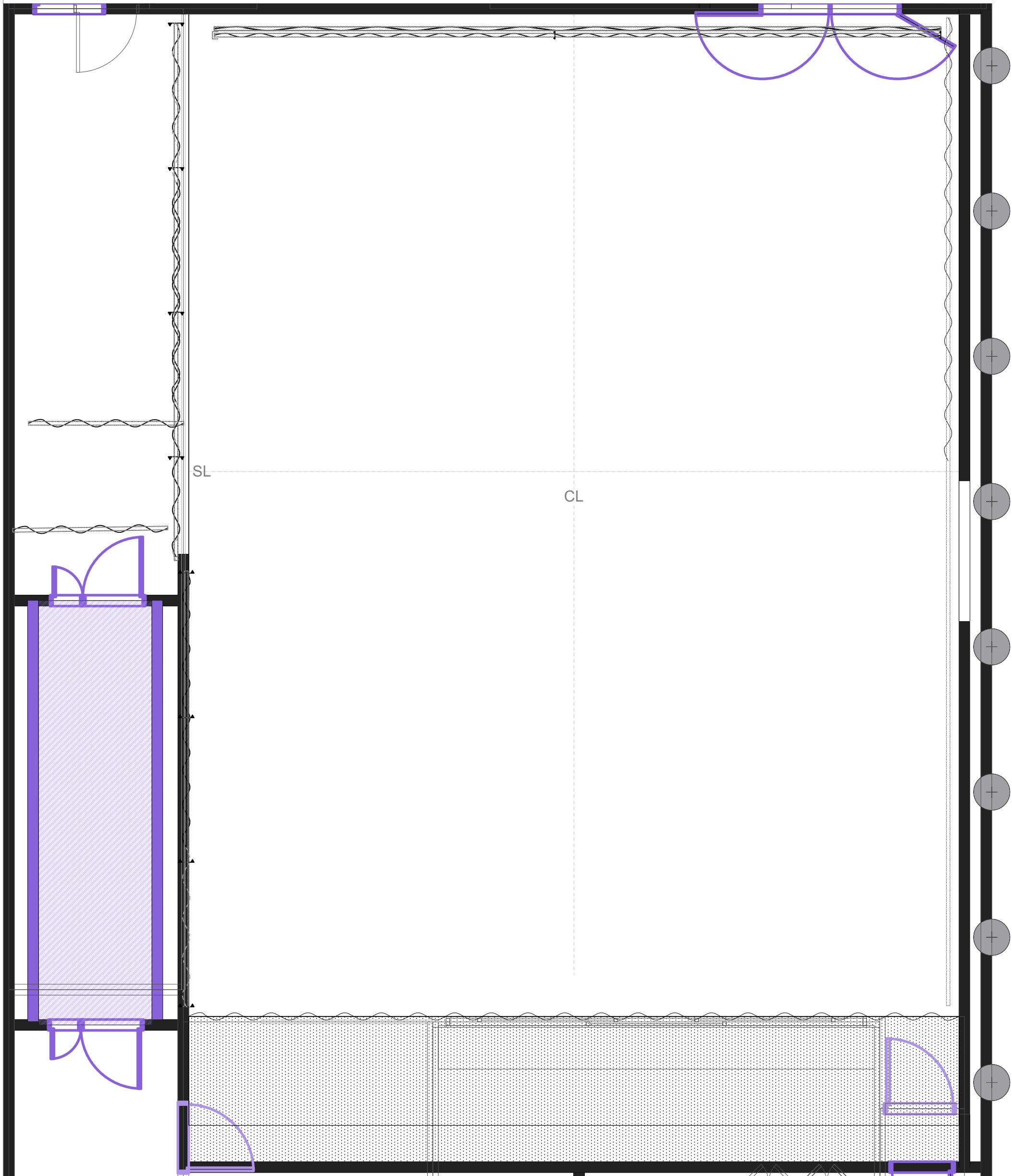
1 NBT_FloorPlan Scale: 1:50
