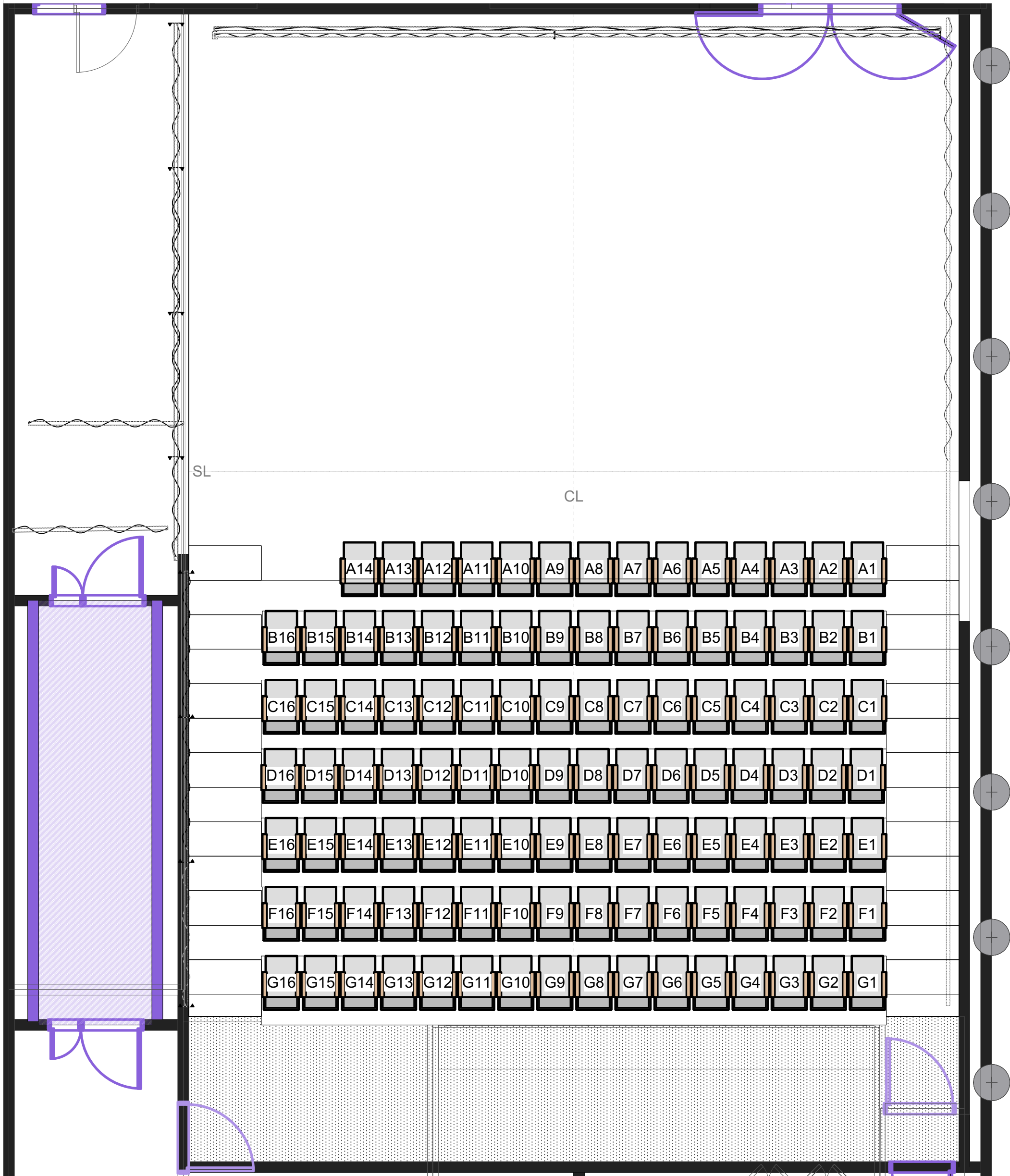
1 NBT_GridPlan Scale: 1:50
