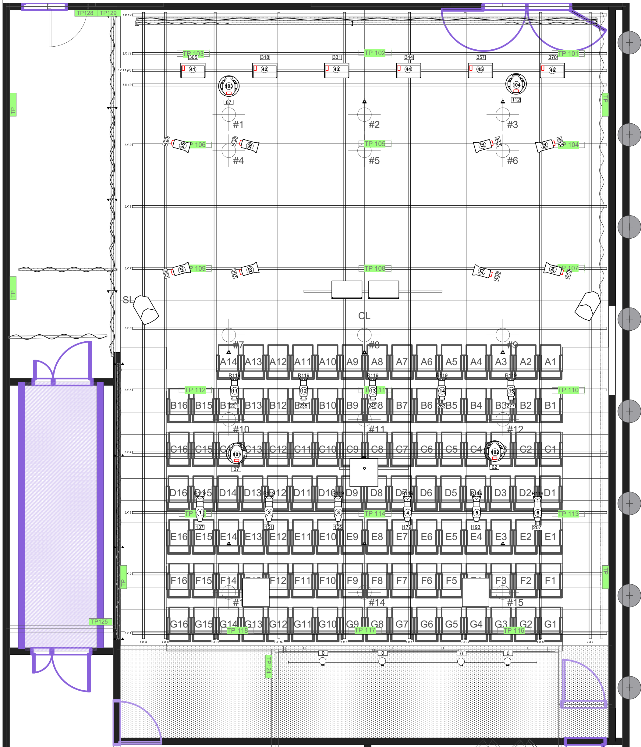
1 NBT_StandardRig Scale: 1:50
