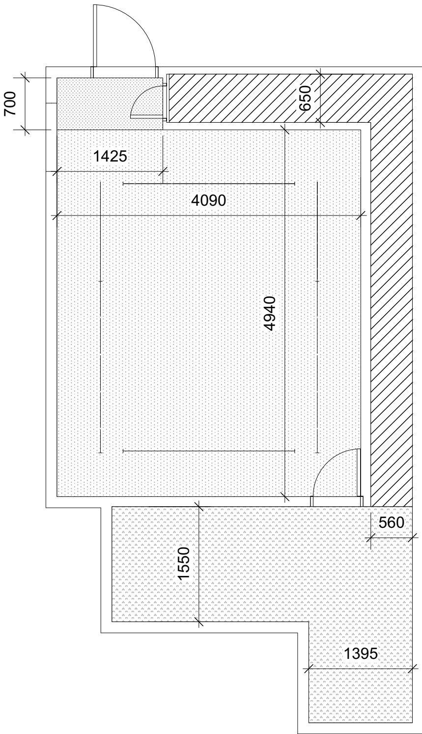
1.1 G2//FloorPlanW/Dimensions Scale: 1:50
