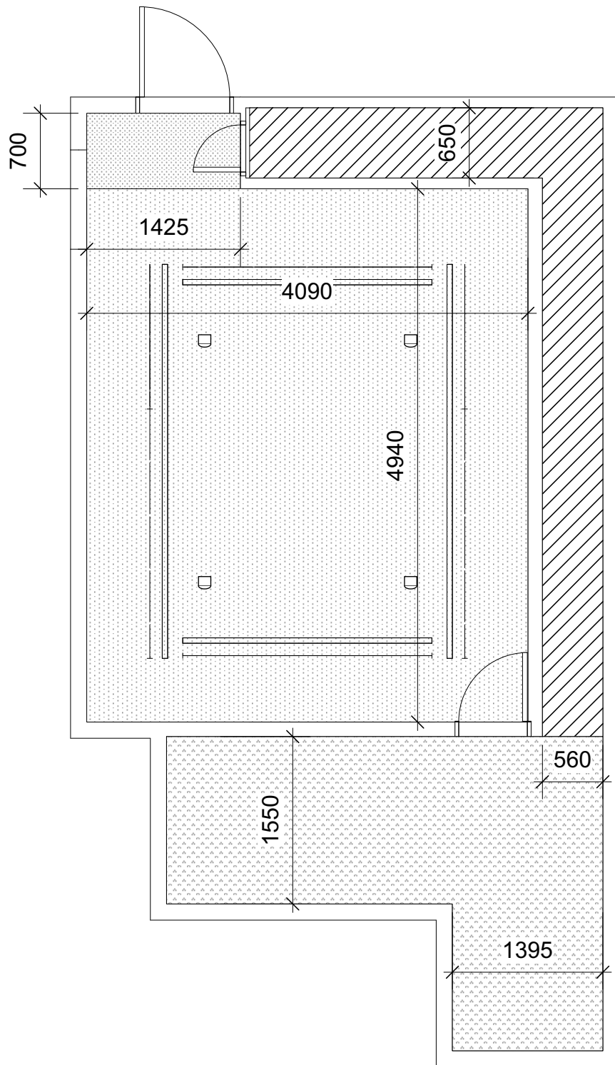
3.1 G2//LightingDimensionsPlan Scale: 1:50
