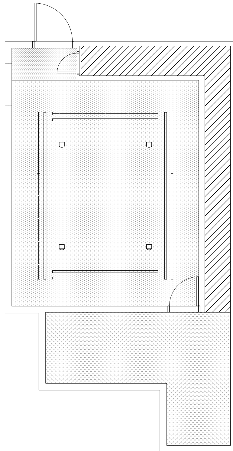
3.0 G2//LightingPlan Scale: 1:50
