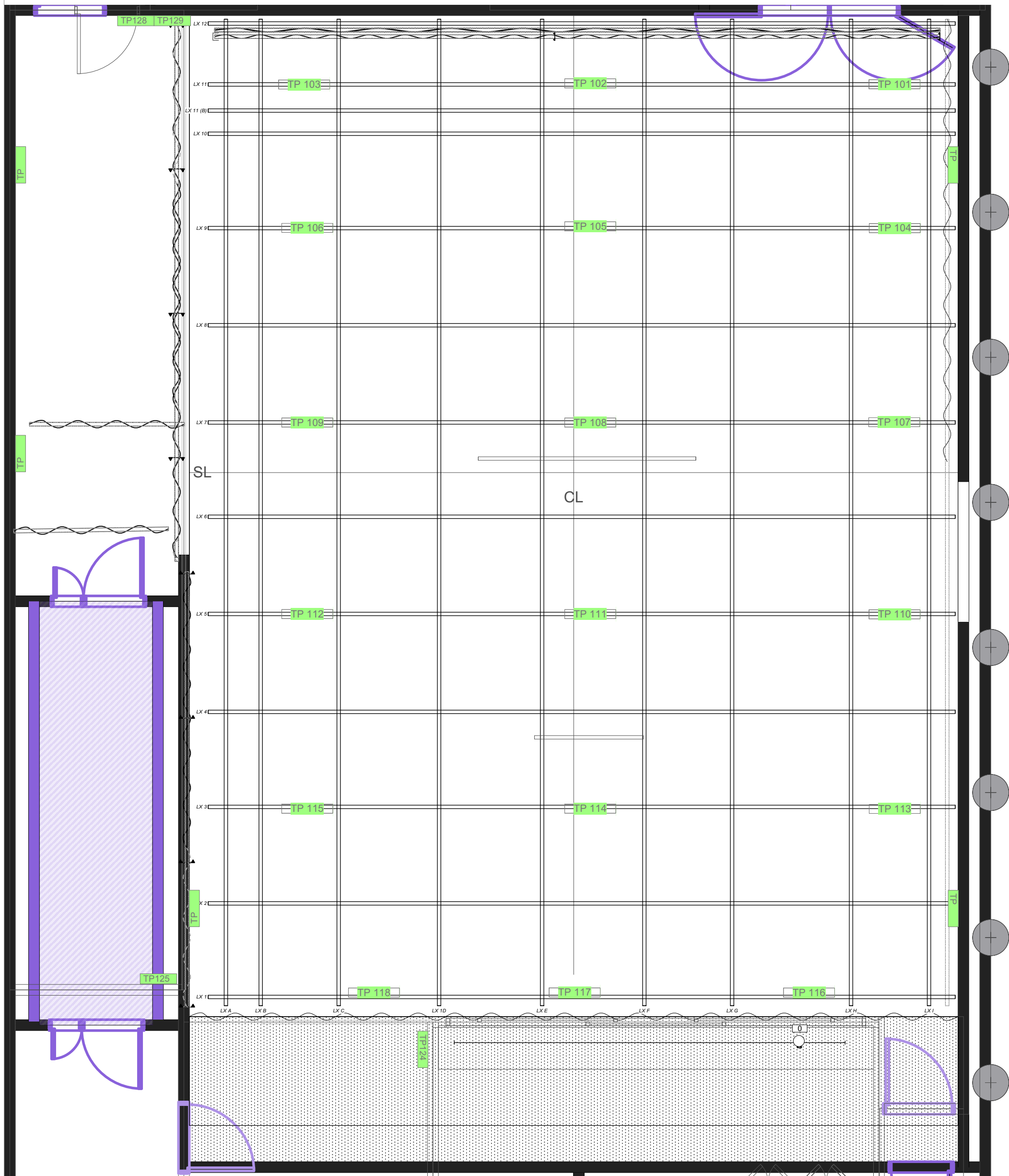
1 NBT_GridPlan Scale: 1:50
